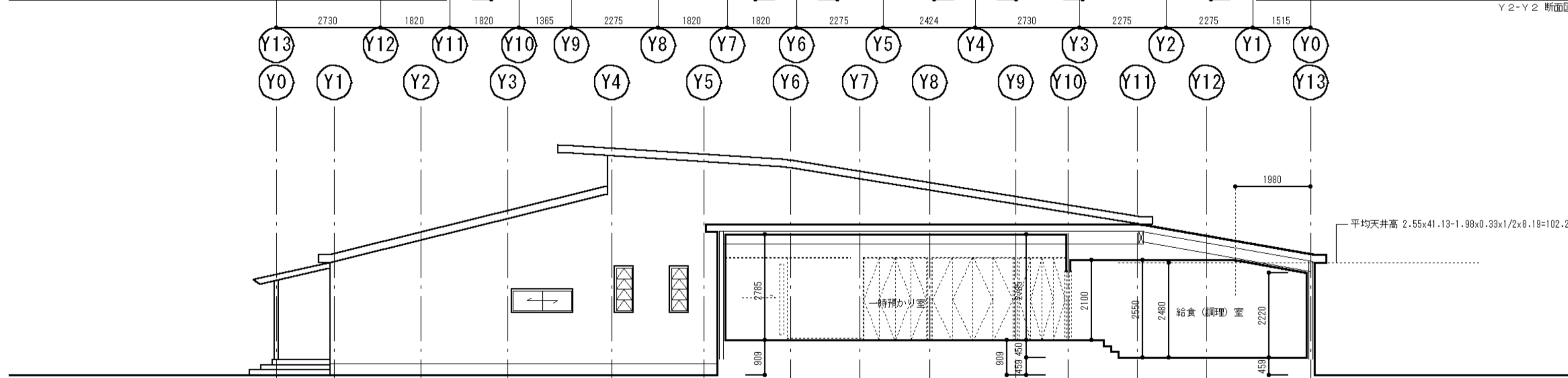
Y3-Y3 断面図
